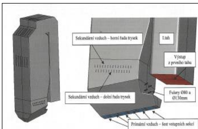
Obr.2.1.1 – Uspořádání kotle, celkový pohled a detail spodní části
