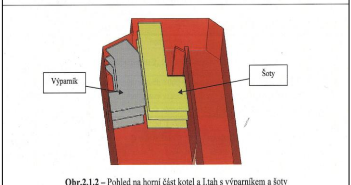
Obr.2.1.2 – Pohled na horní část kotel a I.tah s výparníkem a šoty
