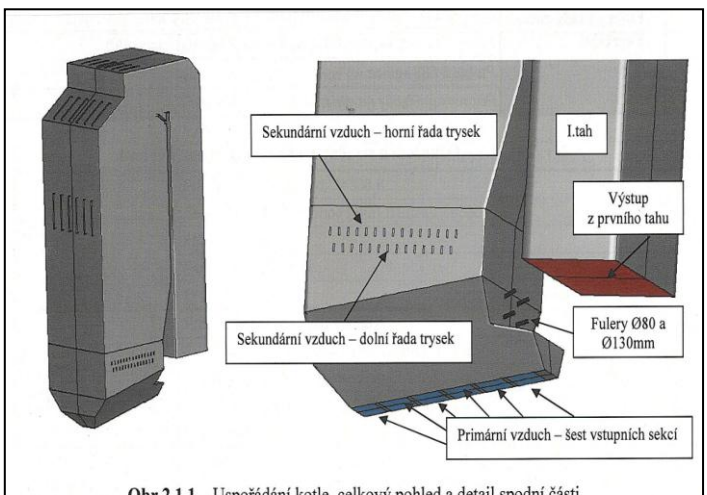
Obr.2.1.1 – Uspořádání kotle, celkový pohled a detail spodní části
